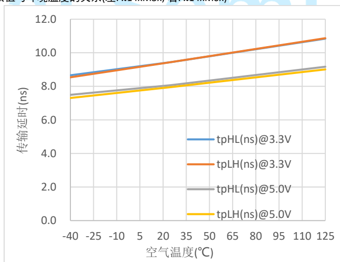
图 8. \pi 14\text{xM}3\text{x} 传输延时 vs. 空气温度
