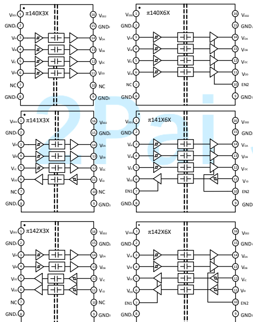
图 1. \pi 140xxx/\pi 141xxx/\pi 142xxx 功能框图
