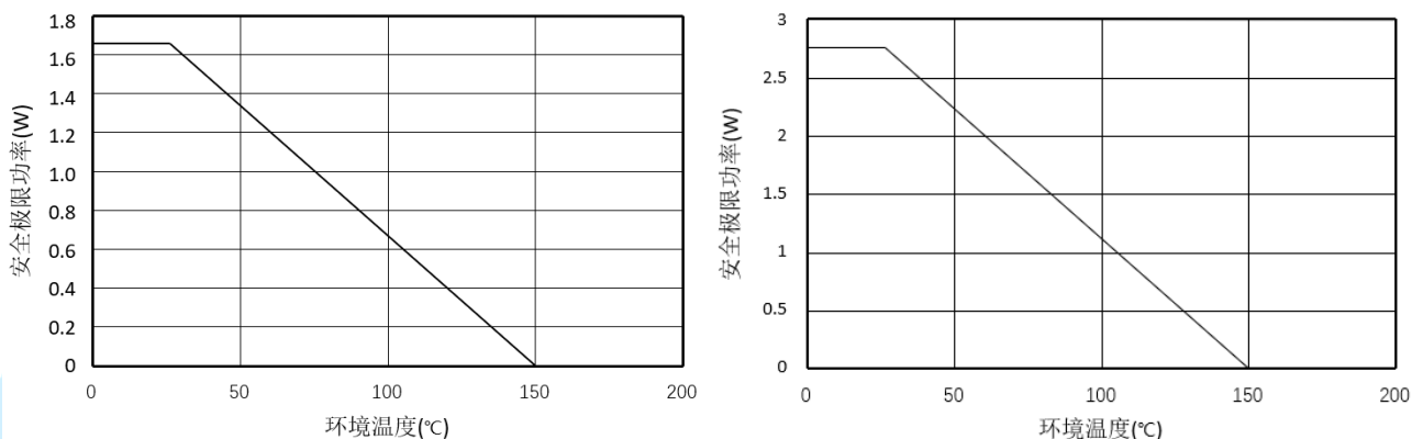
图 6.热降额曲线, 依据 DIN V VDE V 0884-11 的安全限值与环境温度的关系(左: \pi 14\text{xM}3\text{x} ; 右: \pi 14\text{xM}6\text{x} )
