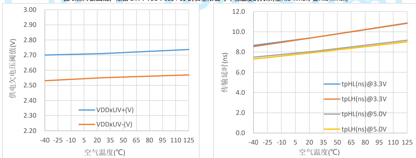
图 7.UVLO vs. 空气温度
