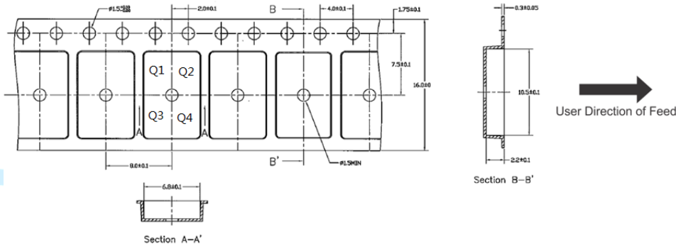
图 22. 16 引脚窄体 SOIC 封装 [NB SOIC-16] 包装信息-尺寸单位(mm)
