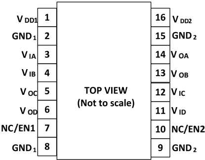
图 5.π142Mxx 管脚定义
