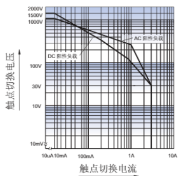
两组常开/常闭触点串联
