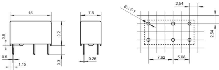
安装孔尺寸 (底视图)
