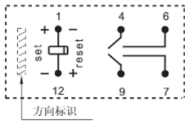
单线圈磁保持
