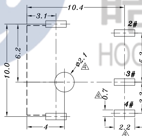
P.C.B LAYOUT
