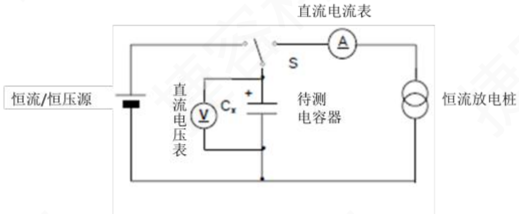
图1 恒流放电方法电路
