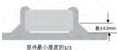
A.回流焊接的最佳焊料用量
