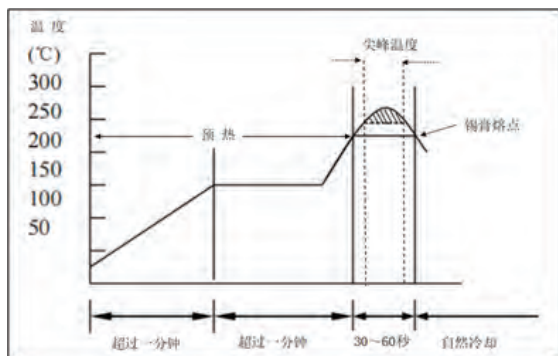
回流焊接
