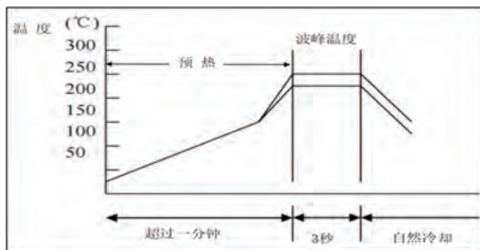
波峰焊接
