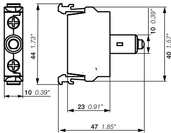
MLBL 尺寸 (mm, 英寸)
