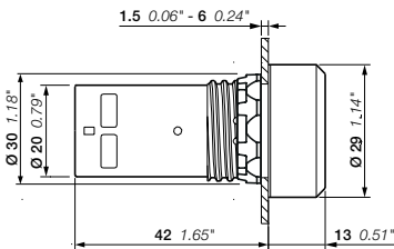
CP1 尺寸 (mm, 英寸)
