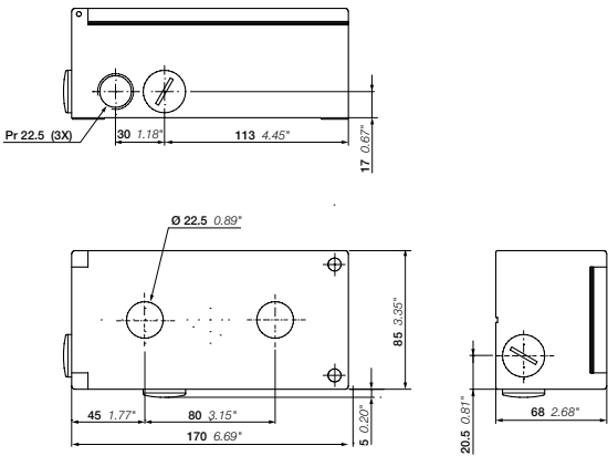
2底座和3底座KEM2-0、KEM3-0
