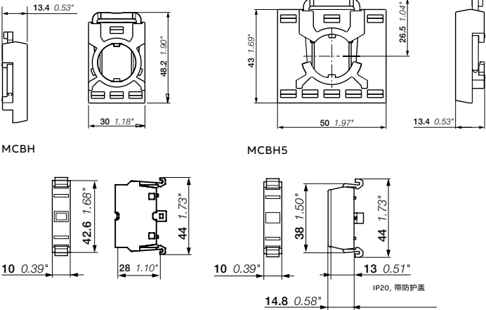
MCBH MCBH5 MCB MCBL 尺寸 (mm, 英寸)
