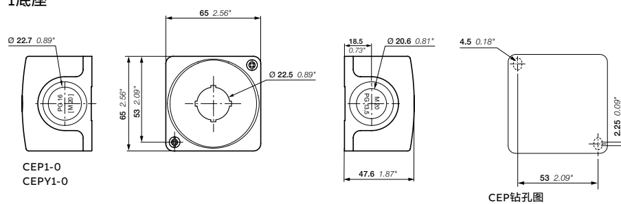
CEP钻孔图
