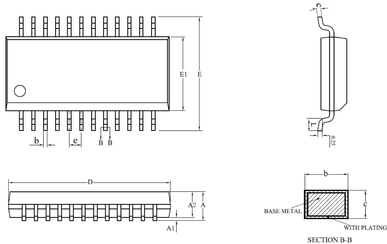
图 3-1 BP32MC057M6S8 封装图示
