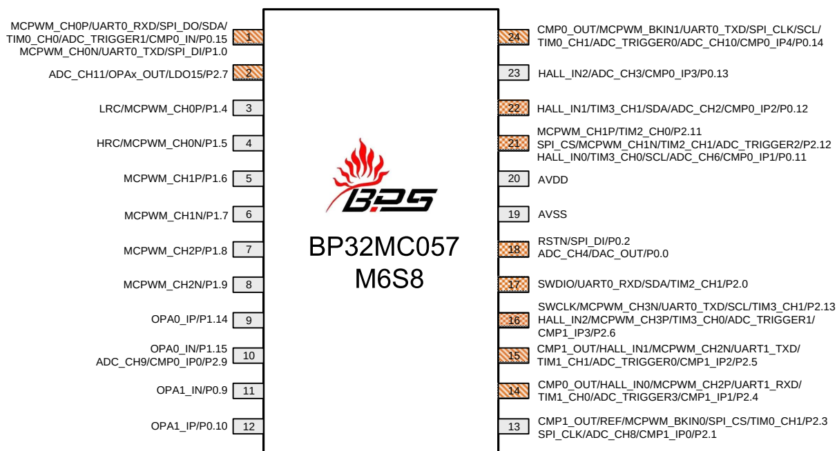
图 2-1 BP32MC057M6S8 管脚分布图
