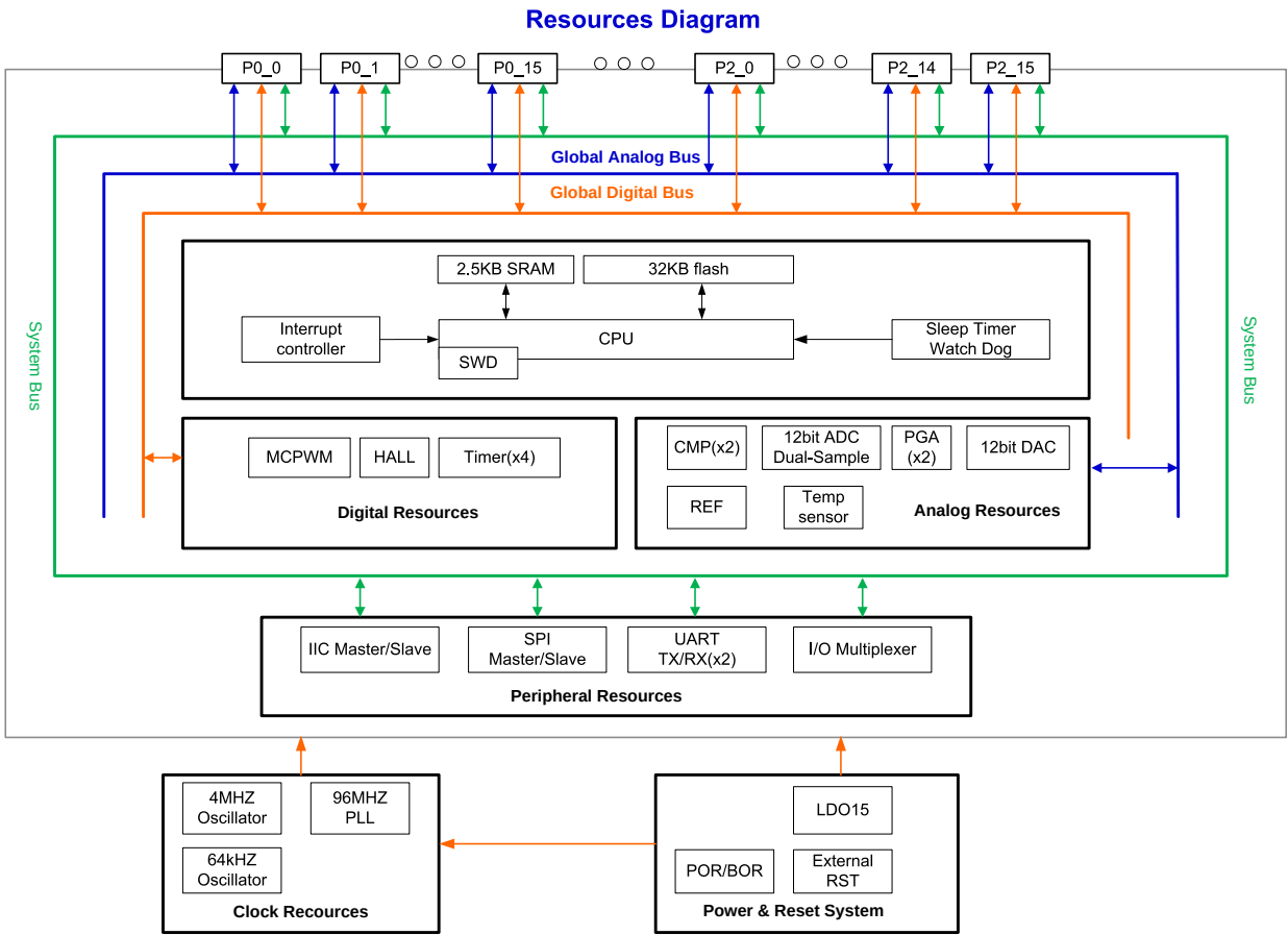
图 1-2 BP32MC057M6S8 系统框图
