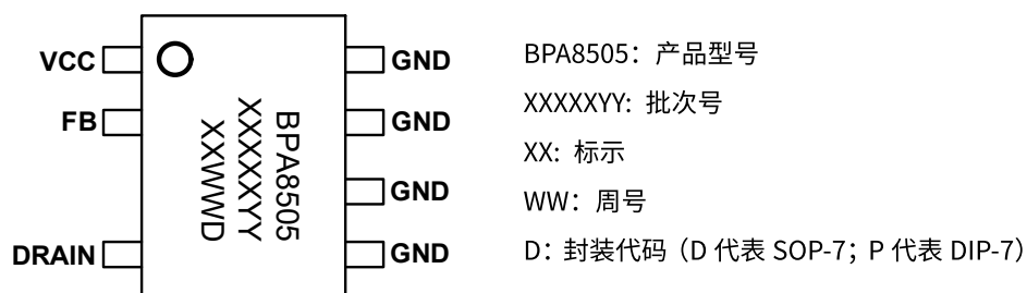
图 2. SOP-7 管脚封装图
