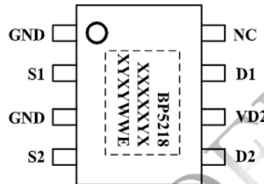
图 2 BP5218E 管脚封装图
