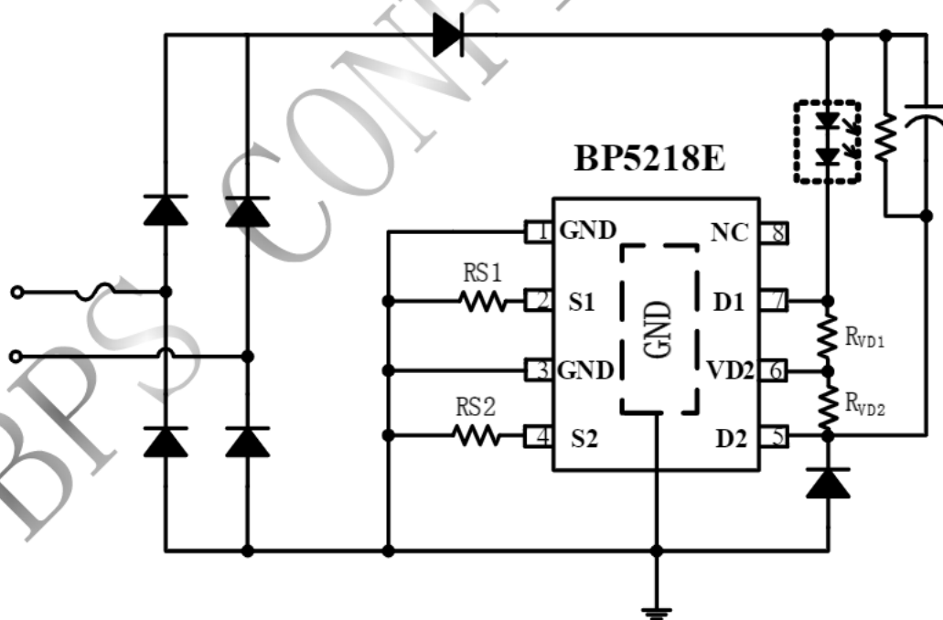
图 1 BP5218E 典型应用图
