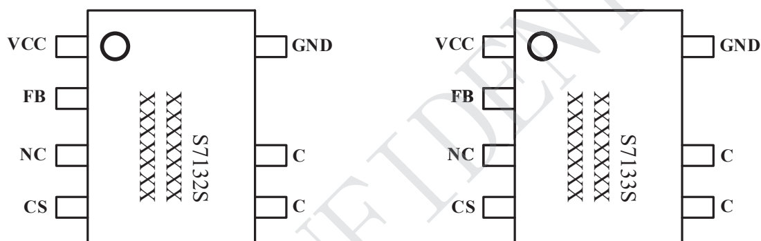
图 2 封装管脚图
