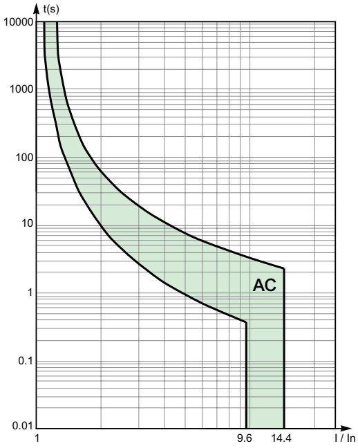
D曲线
