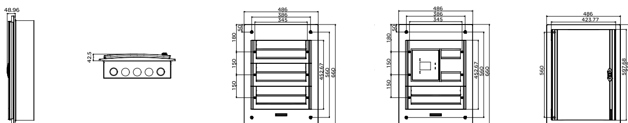
暗装箱 (54位)
