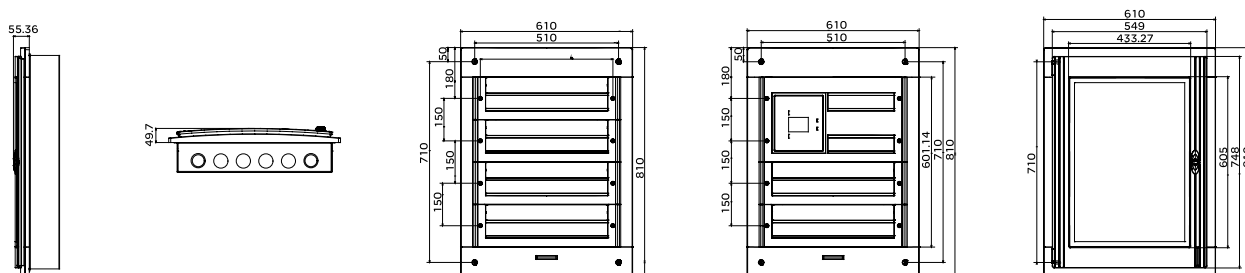
暗装箱 (96位)
