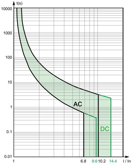
C曲线
