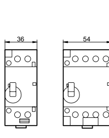
ICT 手动操作接触器 40/63 A
