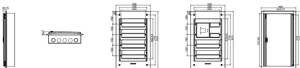
暗装箱 (72位)
