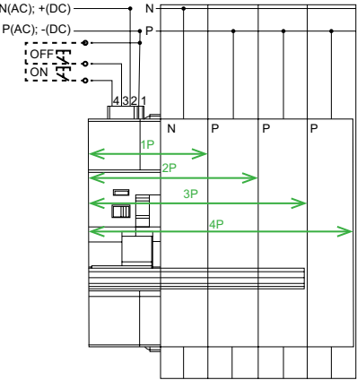
接线图
