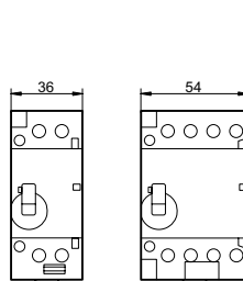
ICT 手动操作接触器 40/63 A
