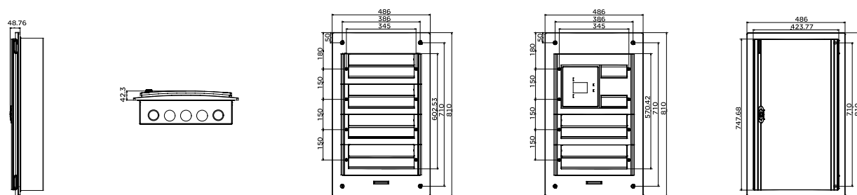
暗装箱 (72位)
