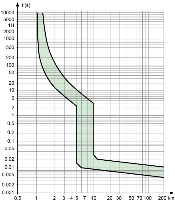
C曲线
