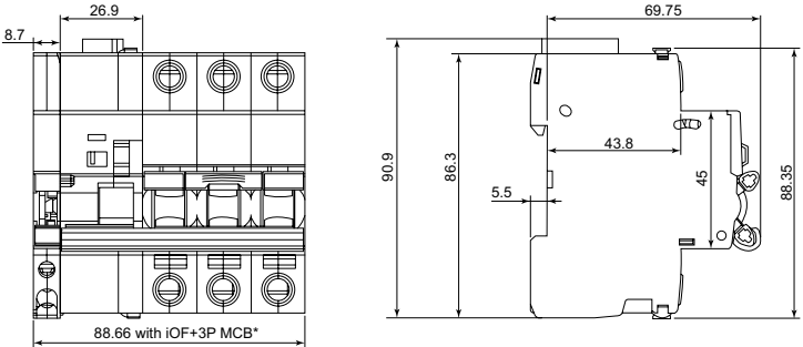
尺寸(mm)
