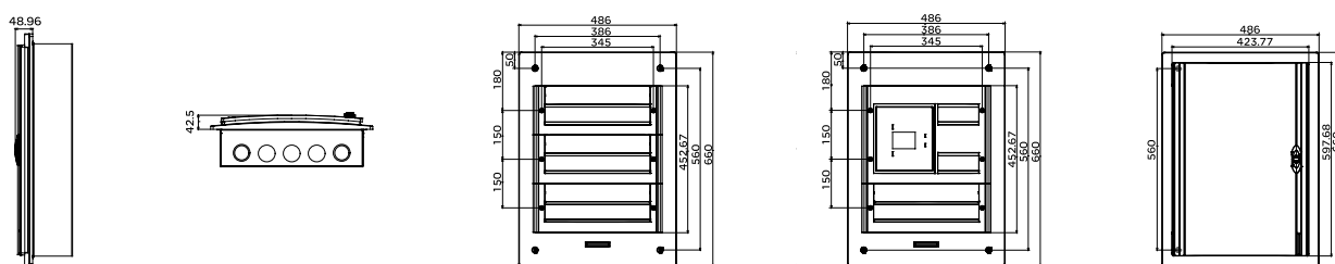
暗装箱 (54位)
