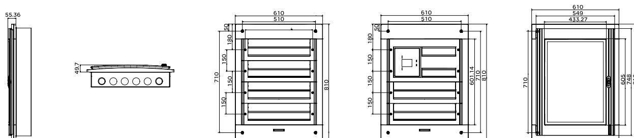
暗装箱 (96位)
