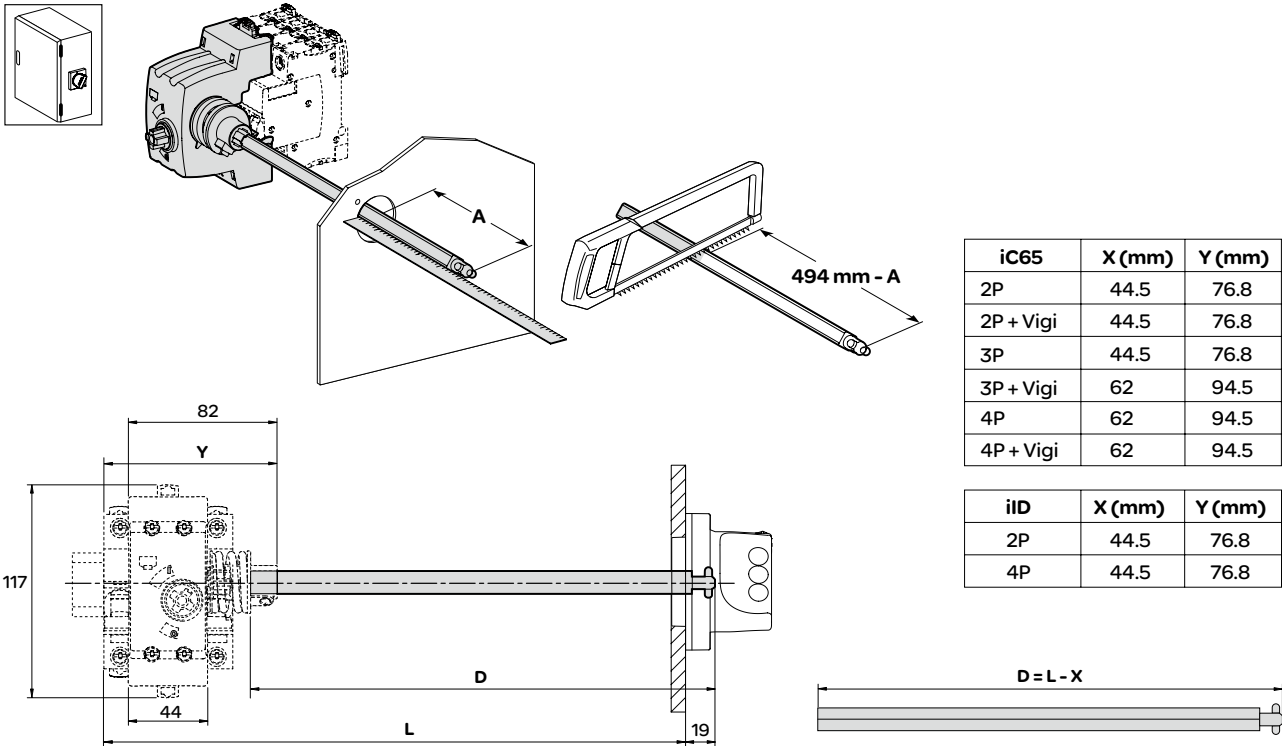
旋转手柄：侧面安装
