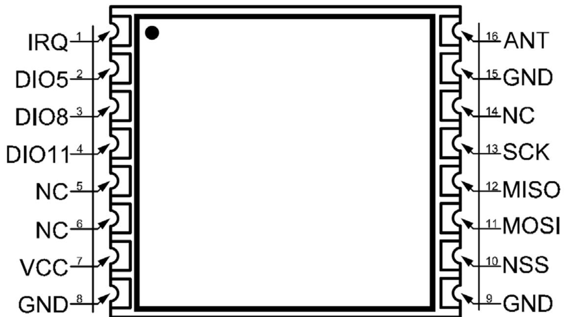
图 3-1 俯视图
