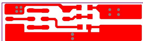
TOP SIDE
