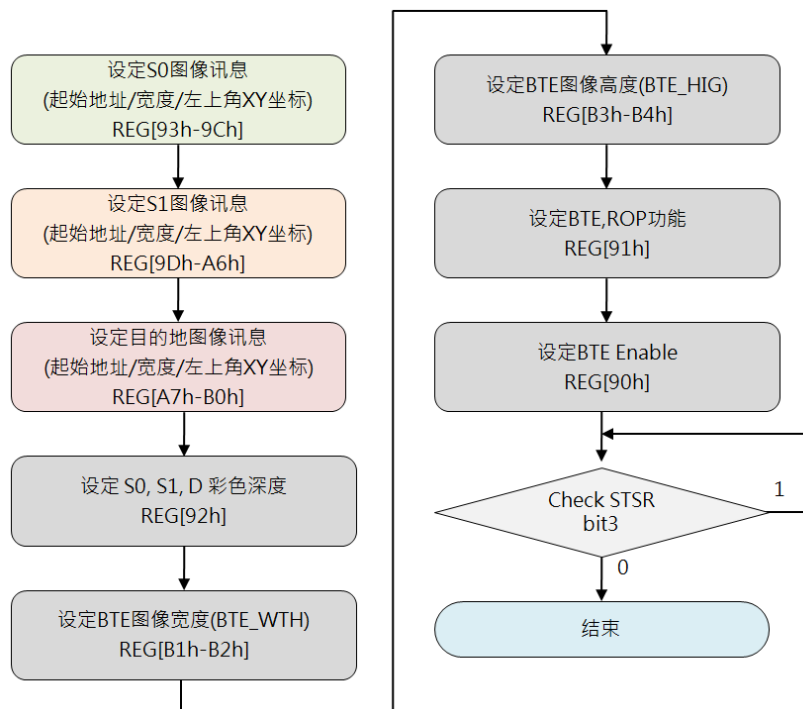
图 15-7: 结合光栅操作的 BTE 内存复制流程图(1)
