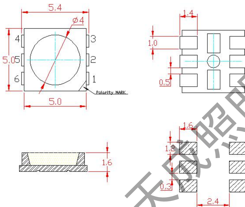
建议焊盘尺寸
