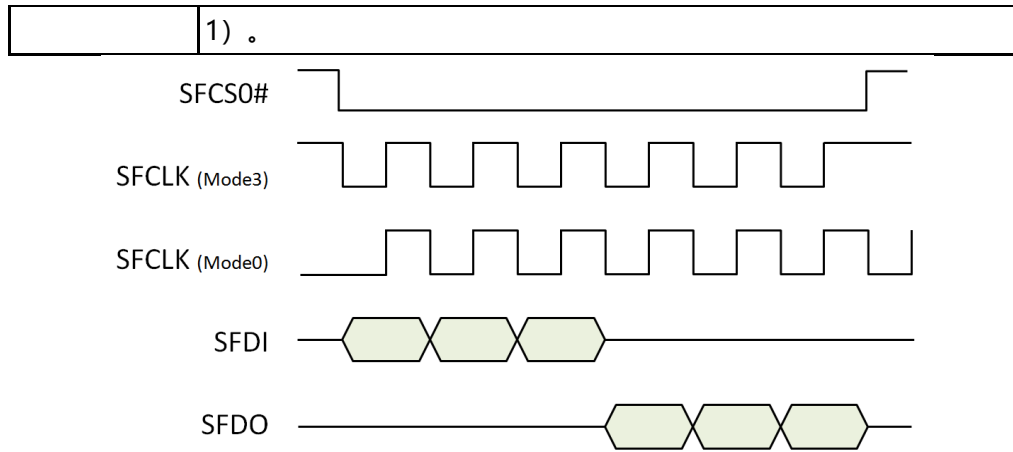
图 15-5: Mode 0 与 Mode3 传输协议
