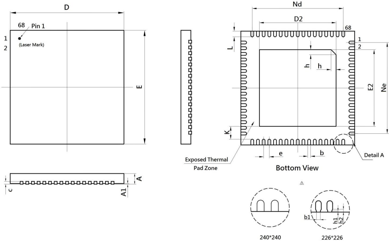
图 19-1: QFN-68Pin 外观尺寸图
