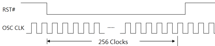
图 6-1: 复位信号
