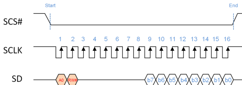
图 7-2: MCU 3 线 SPI 串联界面时序图
