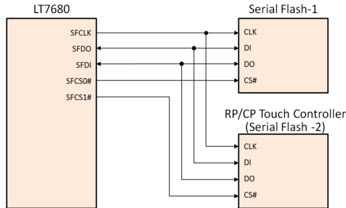
图 15-4: LT7680x-R 串行 Flash/ROM 应用电路
