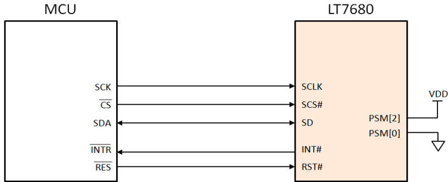
图 7-1: MCU 3 线 SPI 串联接口电路图
