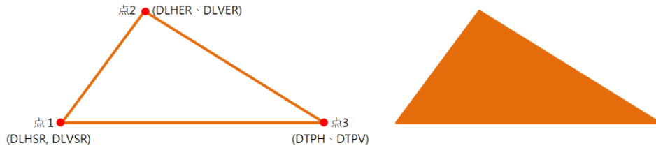
图 11-8: 画三角形
