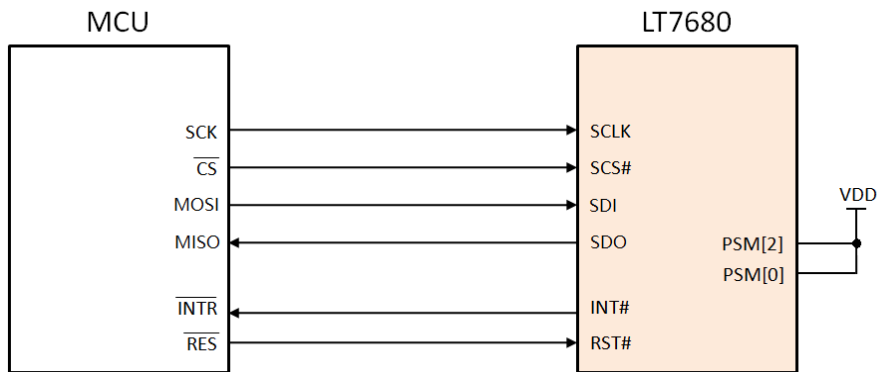
图 7-3: MCU 4 线 SPI 串联接口电路图
