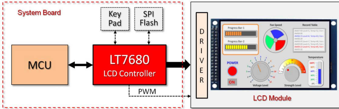
图 1-2: LT7680x-R 设置在系统主板上
