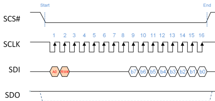
图 7-4: MCU 4 线 SPI 串联界面写入时序图
