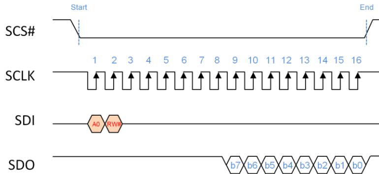
图 7-5: MCU 4 线 SPI 串联接口读取时序图
