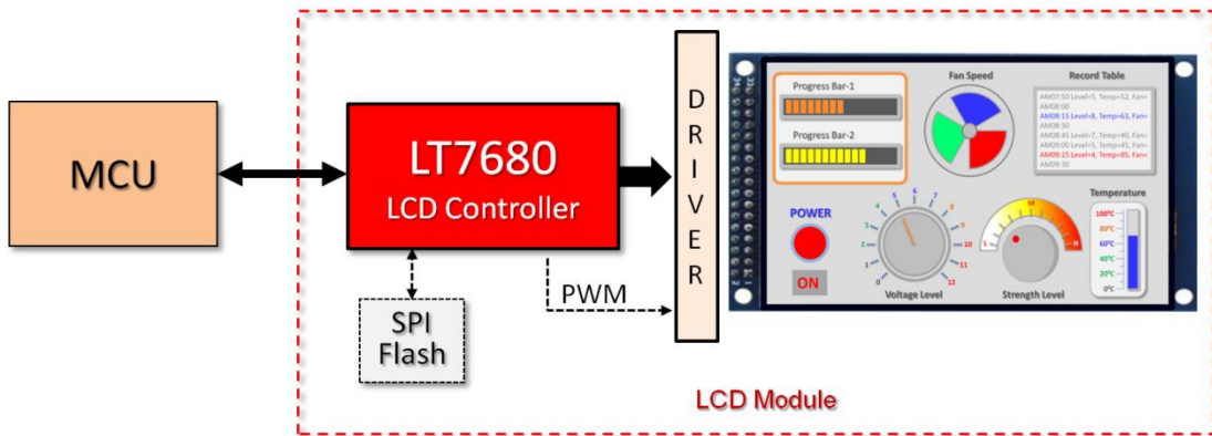
图 1-3: LT7680x-R 设置在 LCD 模块上
