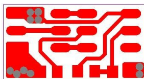
TOP SIDE
