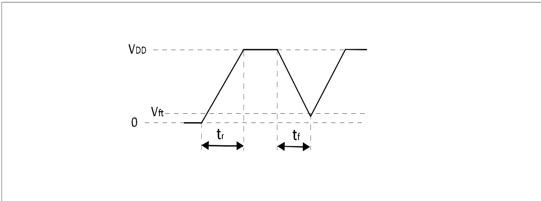
图 13 上电与掉电波形
