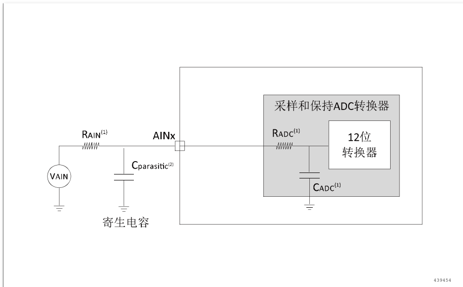
图 24 使用 ADC 典型的连接图
