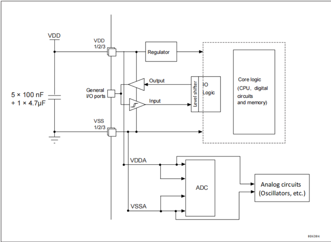
图 11 供电方案
