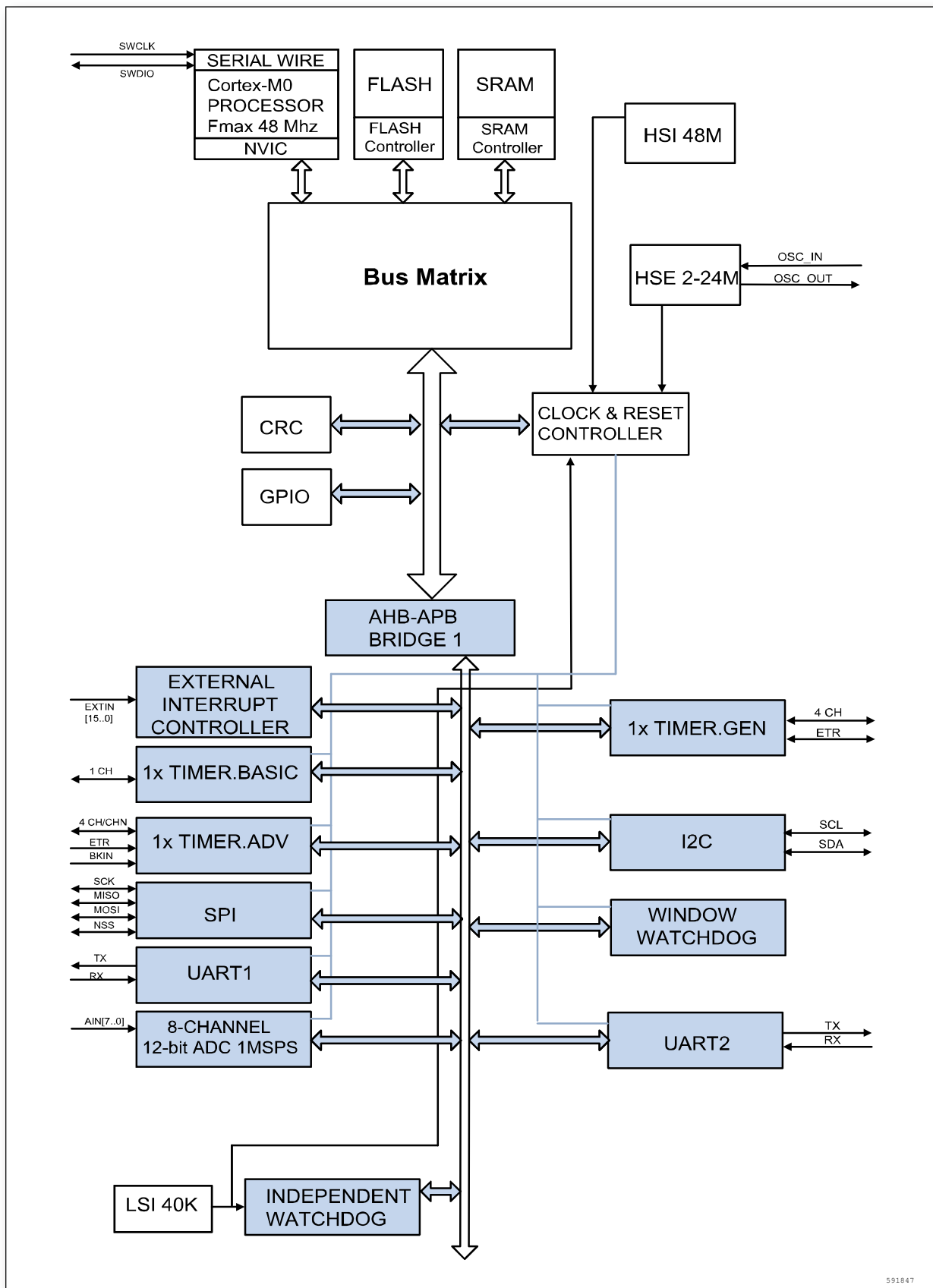
图 4 模块框图
