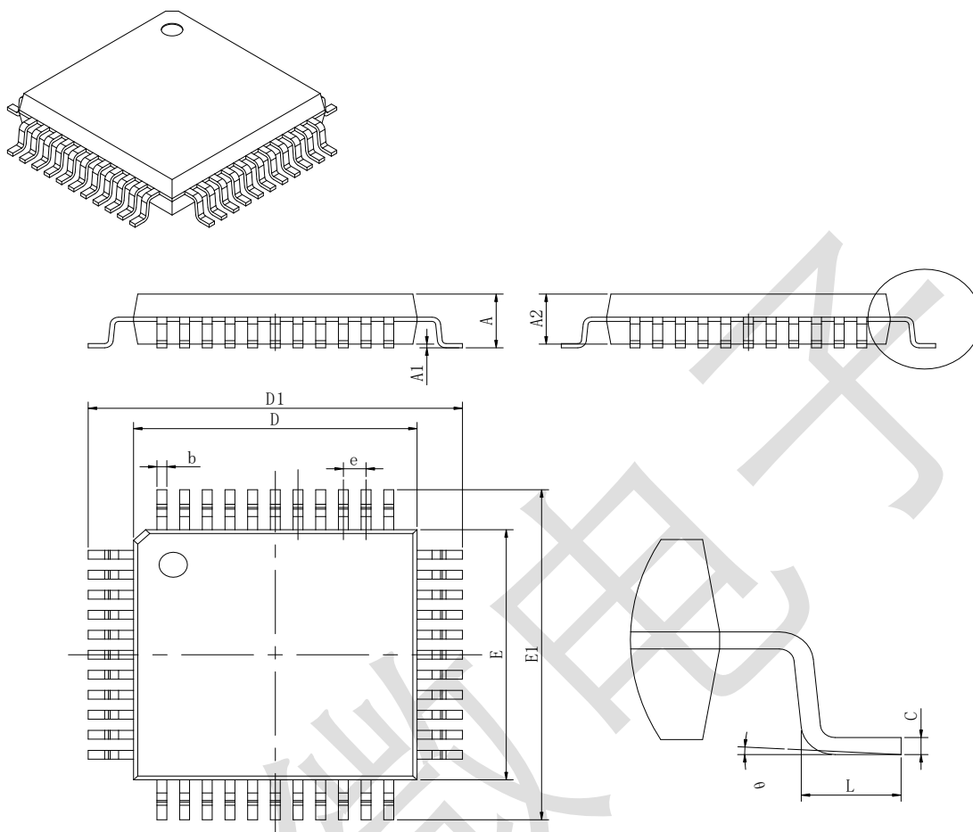
封装示意图 (LQFP44 (短脚) 10mm*10mm)
