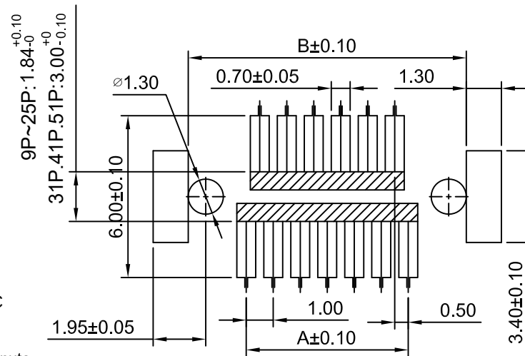
P.C.B YAYOUT
