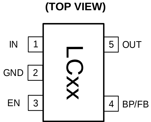
SOT23-5/SOT353(SC70-5)
