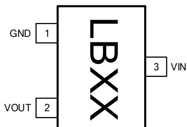
SOT23-3
