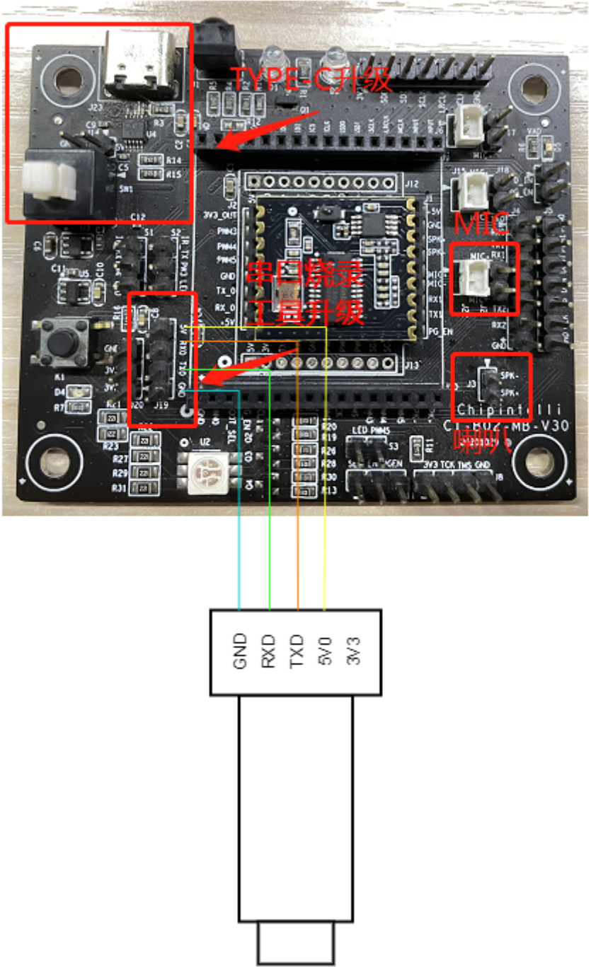
图13 模块和USB转串口工具连接
