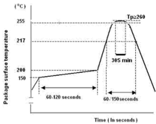
图19 炉温曲线
