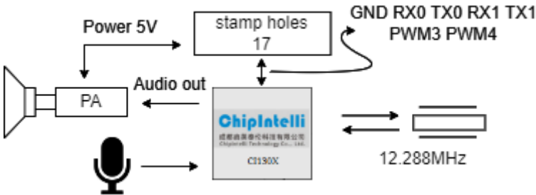
图1 模块框图
