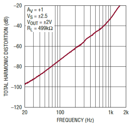
THD 与频率的关系
