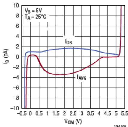
输入失调和平均电流与输入共模电压的关系
