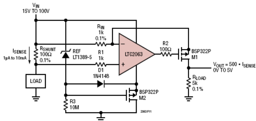
图 11. 高端电流检测
