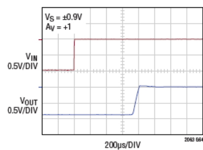
负输入过载恢复
