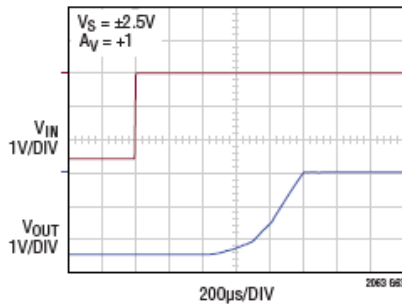
负输入过载恢复
