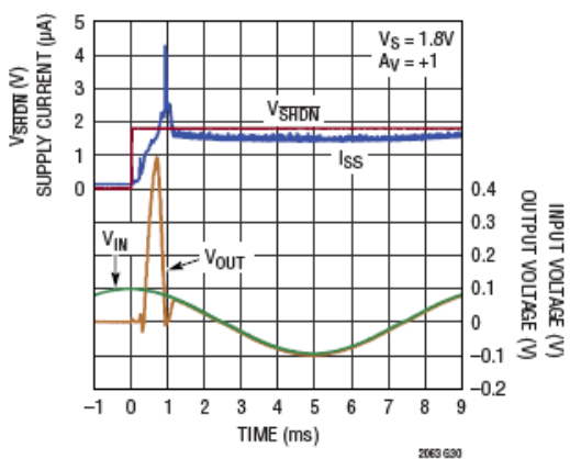
正弦输入的使能瞬变
