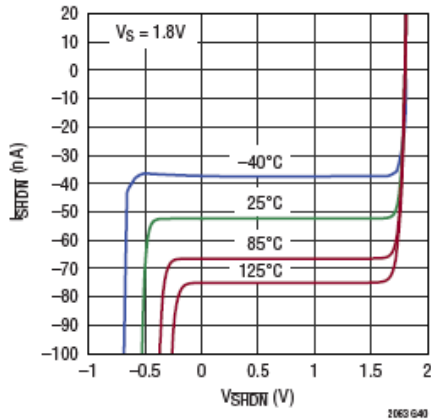
SHDN 引脚上拉电流与 SHDN 引脚电压的关系
