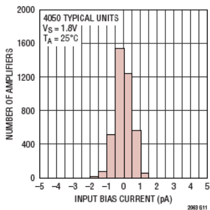
输入偏置电流分布
