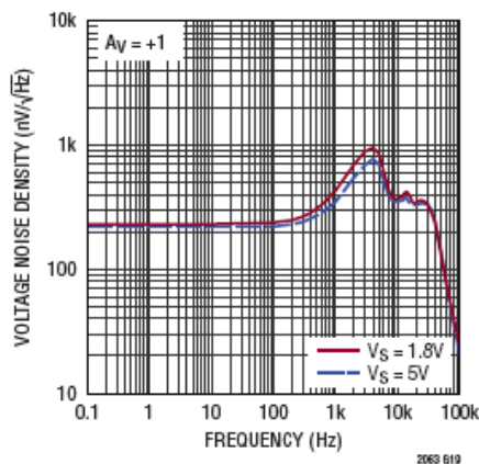
折合到输入端电压噪声密度
