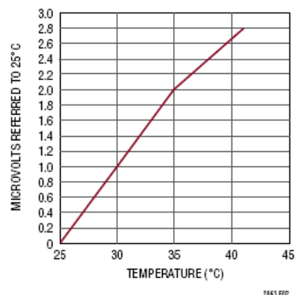
图 2. 不同厂家生产的两条铜线产生的热电动势
