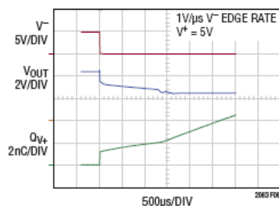
图 6. 上电期间的电荷损失
