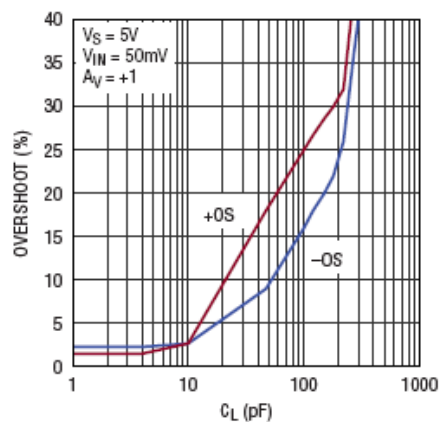
小信号过冲与负载电容的关系
