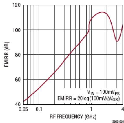
EMI 抑制与频率的关系
