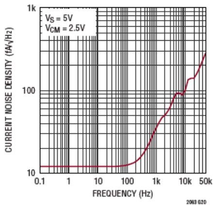
折合到输入端电流噪声密度
