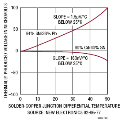
图 3. 焊料-铜热电动势
