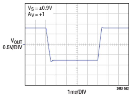
大信号响应
