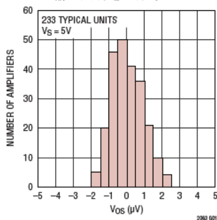
输入失调电压分布
