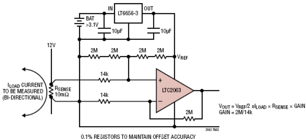
电池供电电流检测电路随同检测电阻电压浮空
