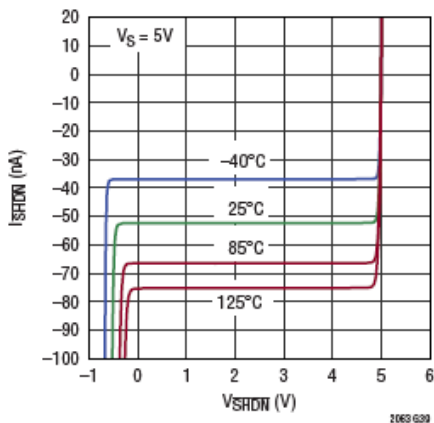
SHDN 上拉电流与 SHDN 引脚电压的关系
