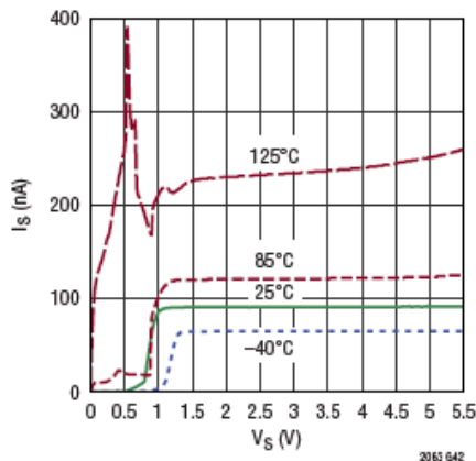
关断电源电流与电源电压的关系
