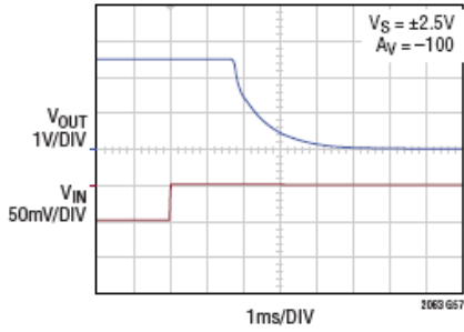
正输出过载恢复
