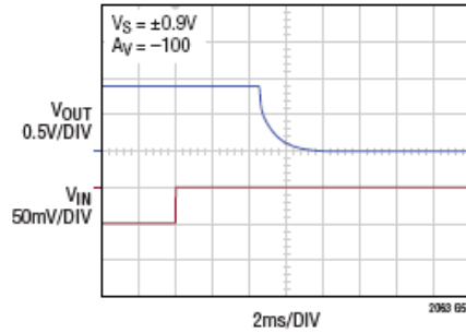
正输出过载恢复
