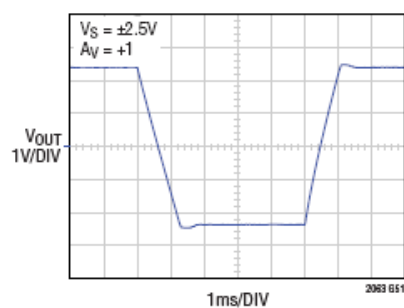
大信号响应
