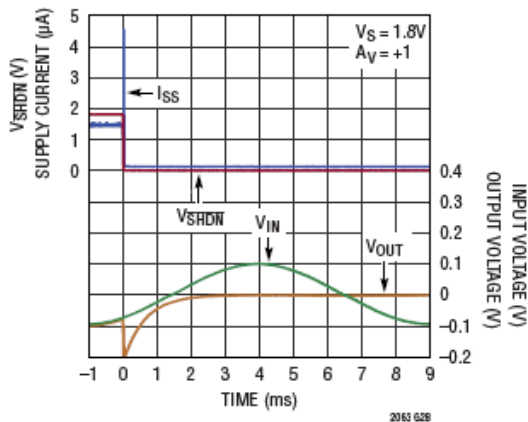
正弦输入的关断瞬变
