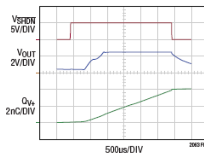
图 7. 通过 \overline{\text{SHDN}} 引脚使能和禁用所导致的电荷损失
