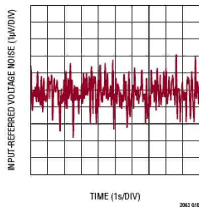
DC 至 10Hz 电压噪声
