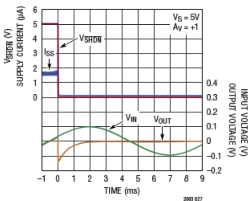
正弦输入的关断瞬变
