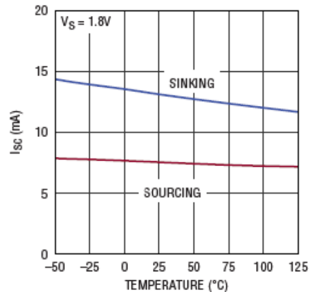
输出短路电流与温度的关系
