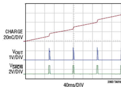
占空比降低系统功耗
