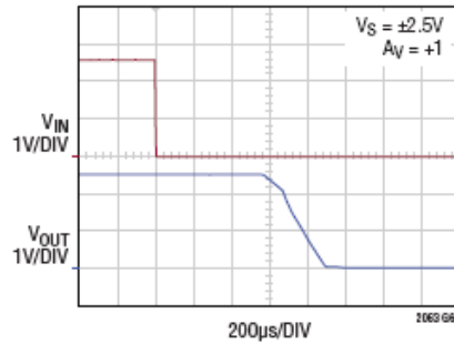
正输入过载恢复
