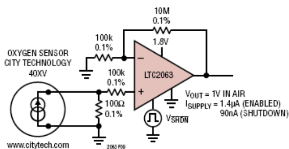
图 9. 低功耗精密氧传感器
