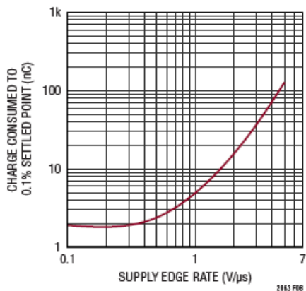
图 8. 上电电荷与电源边沿速率的关系
