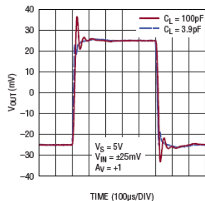
小信号响应
