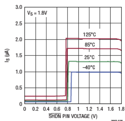
电源电流与 SHDN 引脚电压的关系
