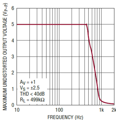
最大无失真输出幅值与频率的关系
