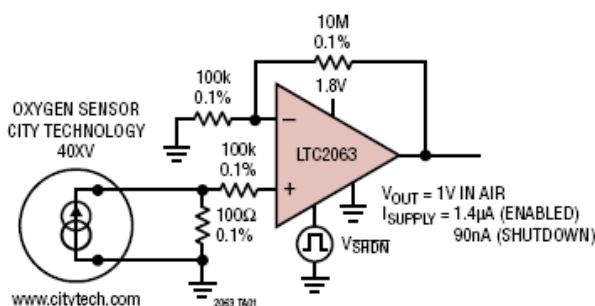
低功耗精密氧传感器
