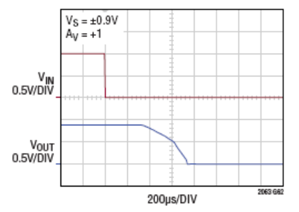
正输入过载恢复
