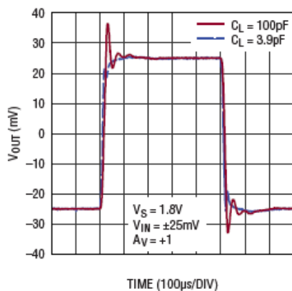
小信号响应
