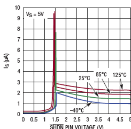
电源电流与 SHDN 引脚电压的关系
