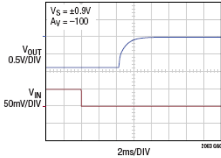
负输出过载恢复
