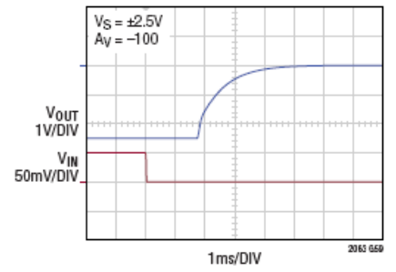
负输出过载恢复
