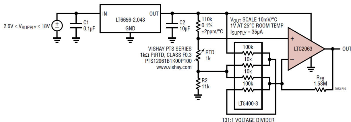
图 10. RTD 传感器
