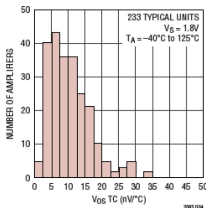
输入失调电压漂移分布
