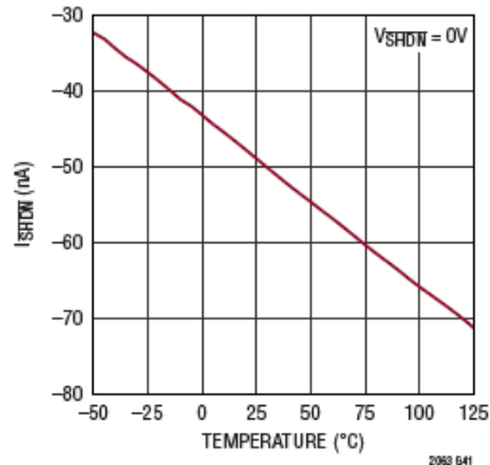
SHDN 引脚电流与温度的关系
