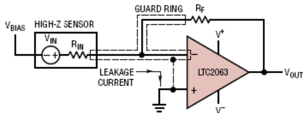
图 5. 带漏电保护环的反相放大器的布局示例
