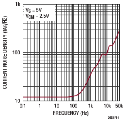
图 1. 输入电流噪声谱
