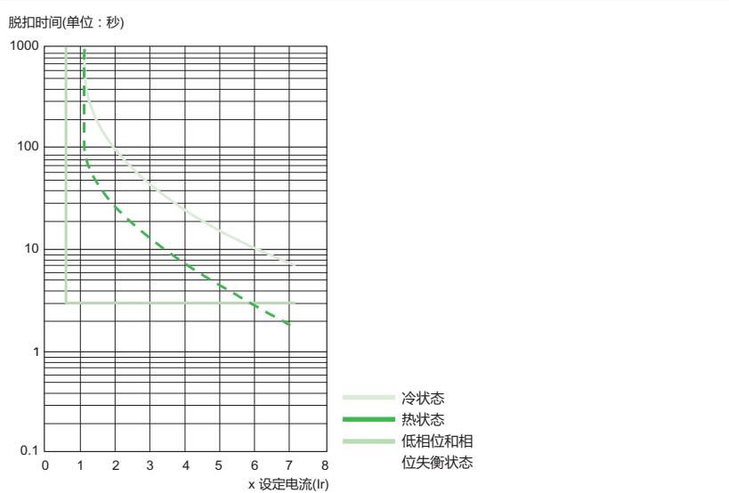
类别 30 的脱扣曲线
