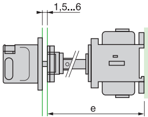
加长轴
