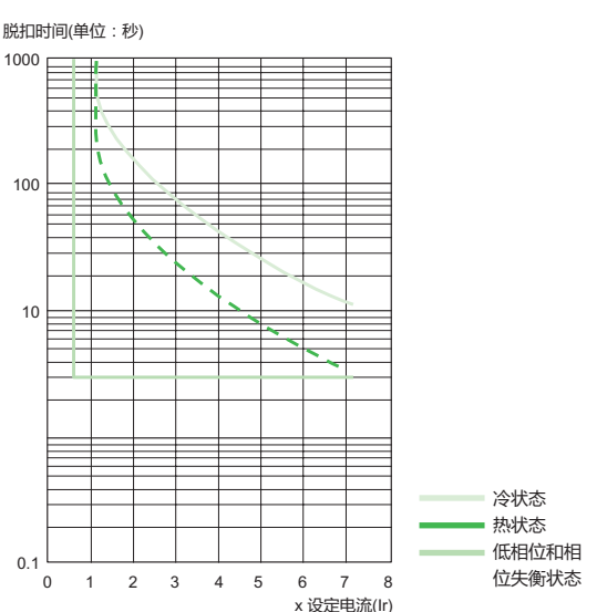
类别 20 的脱扣曲线
