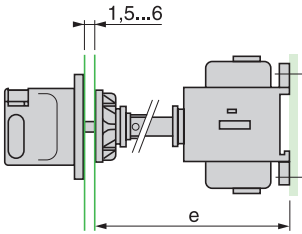
距离 (e) 柜体后部 / 门 mm
