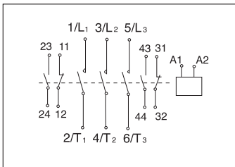
CDC10-20, 40接线图
