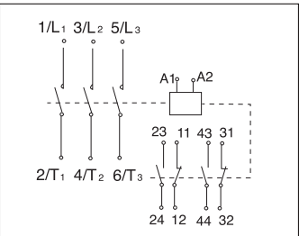
CDC10-60, 100, 150接线图
