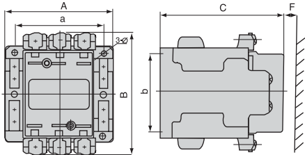
图2 CDC10-20, 40外形及安装尺寸
