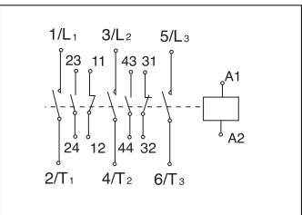
CDC10-10接线图
