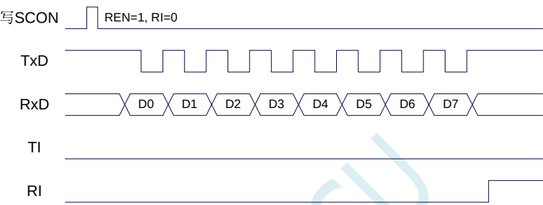
接收数据（串口1模式0）
