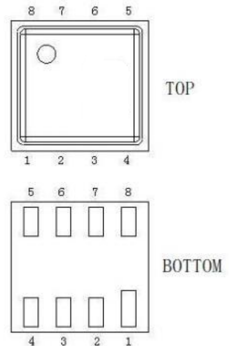
图 2: 引脚图
