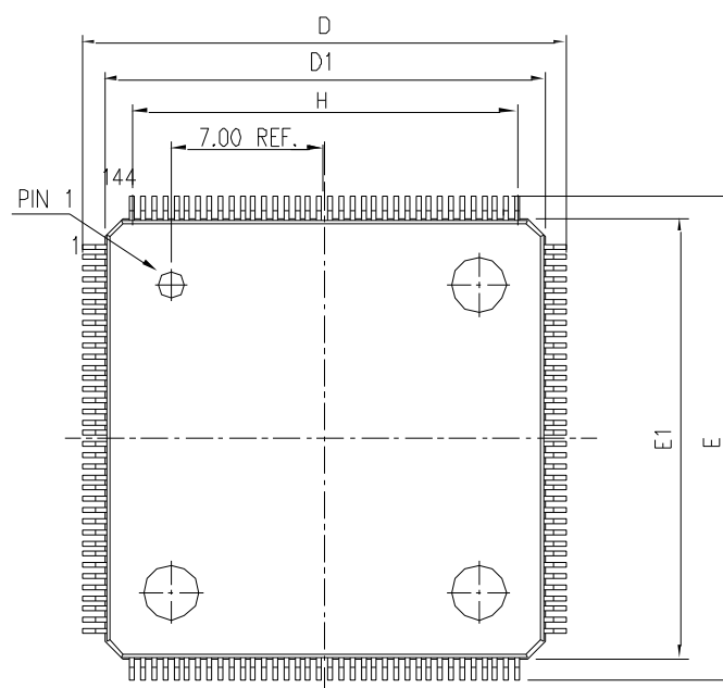
图 20 LQFP144 封装图
