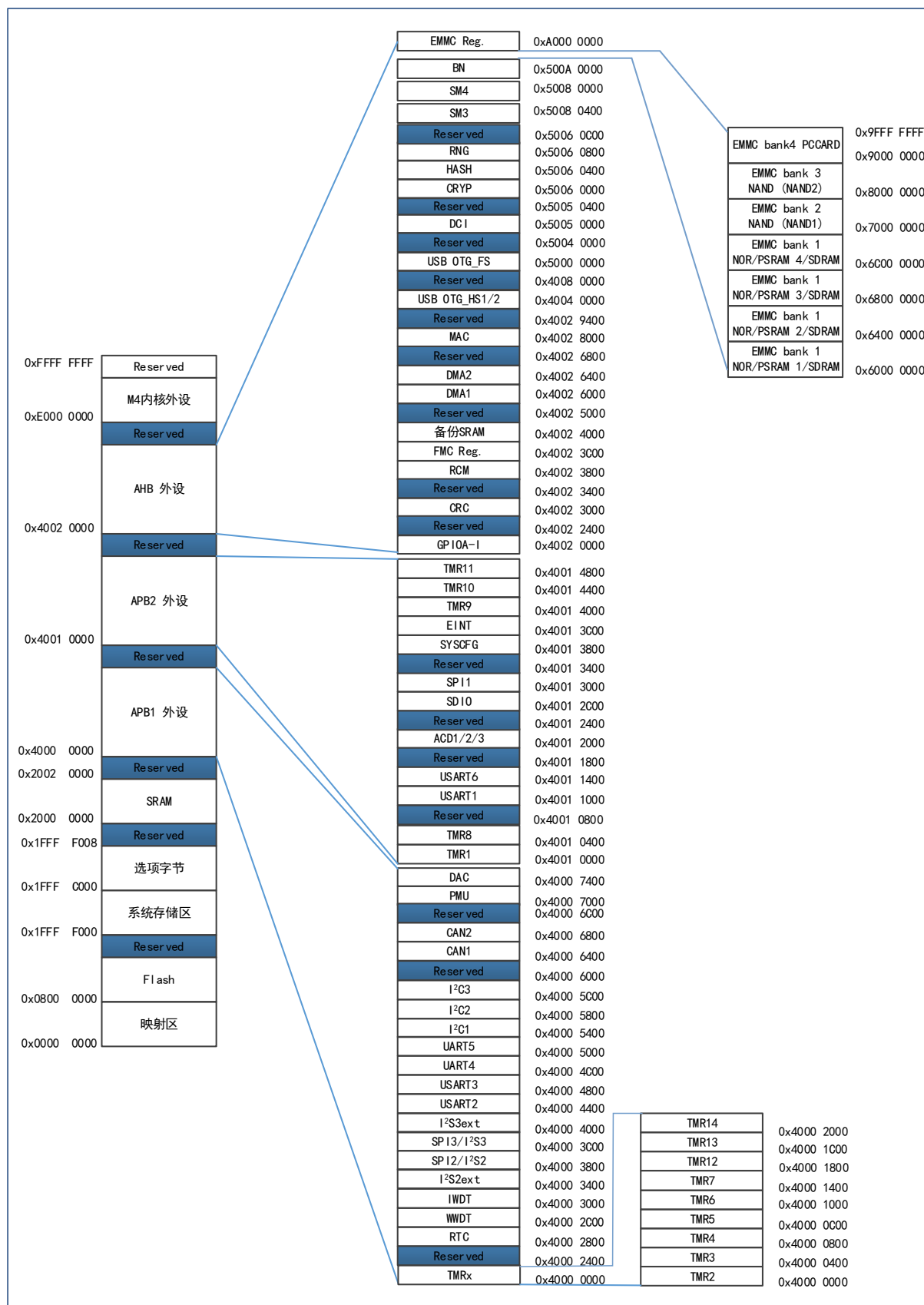
图 6 APM32F415xG 417xExG 系列地址映射图
