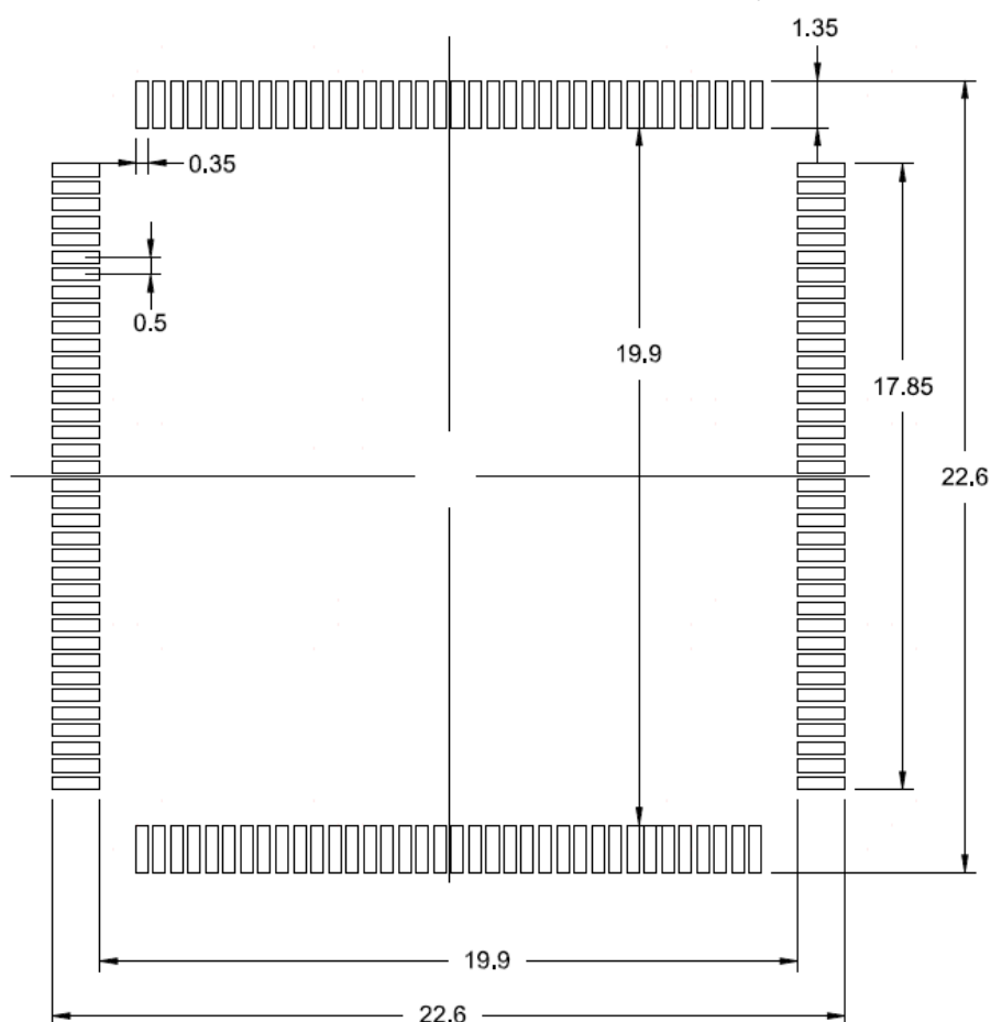
图 22 LQFP144 -144 引脚, 20 x20mm 示意图
