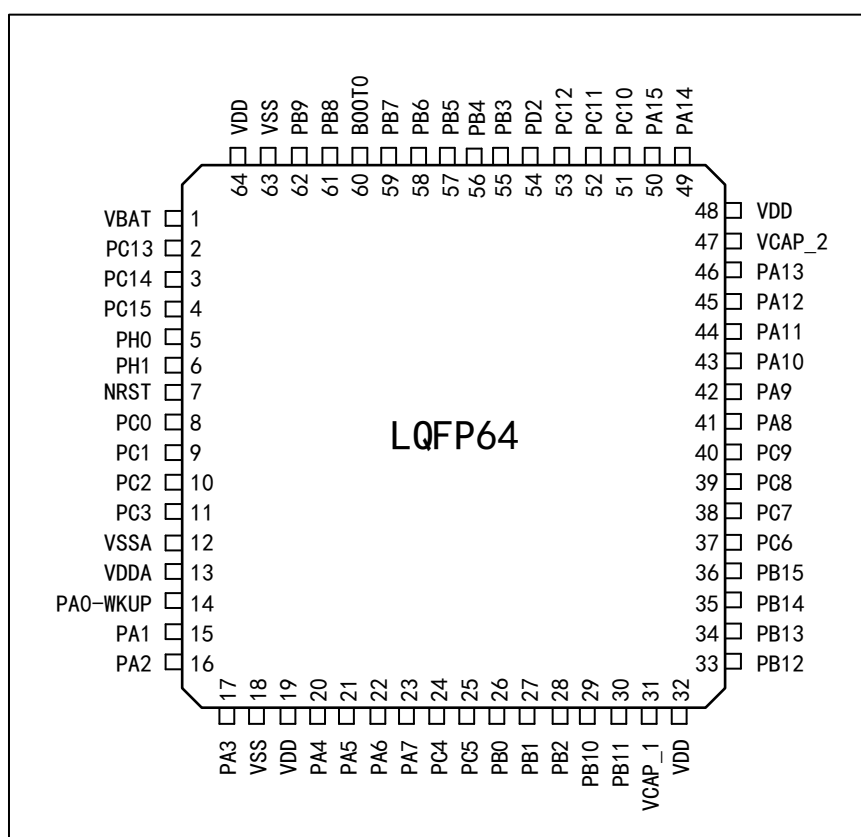
图 4 APM32F415xG 系列 LQFP64 引脚分布图
