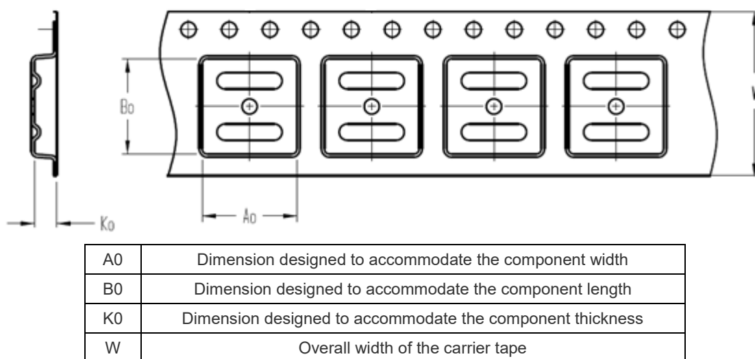
图 29 带状包装规格图
