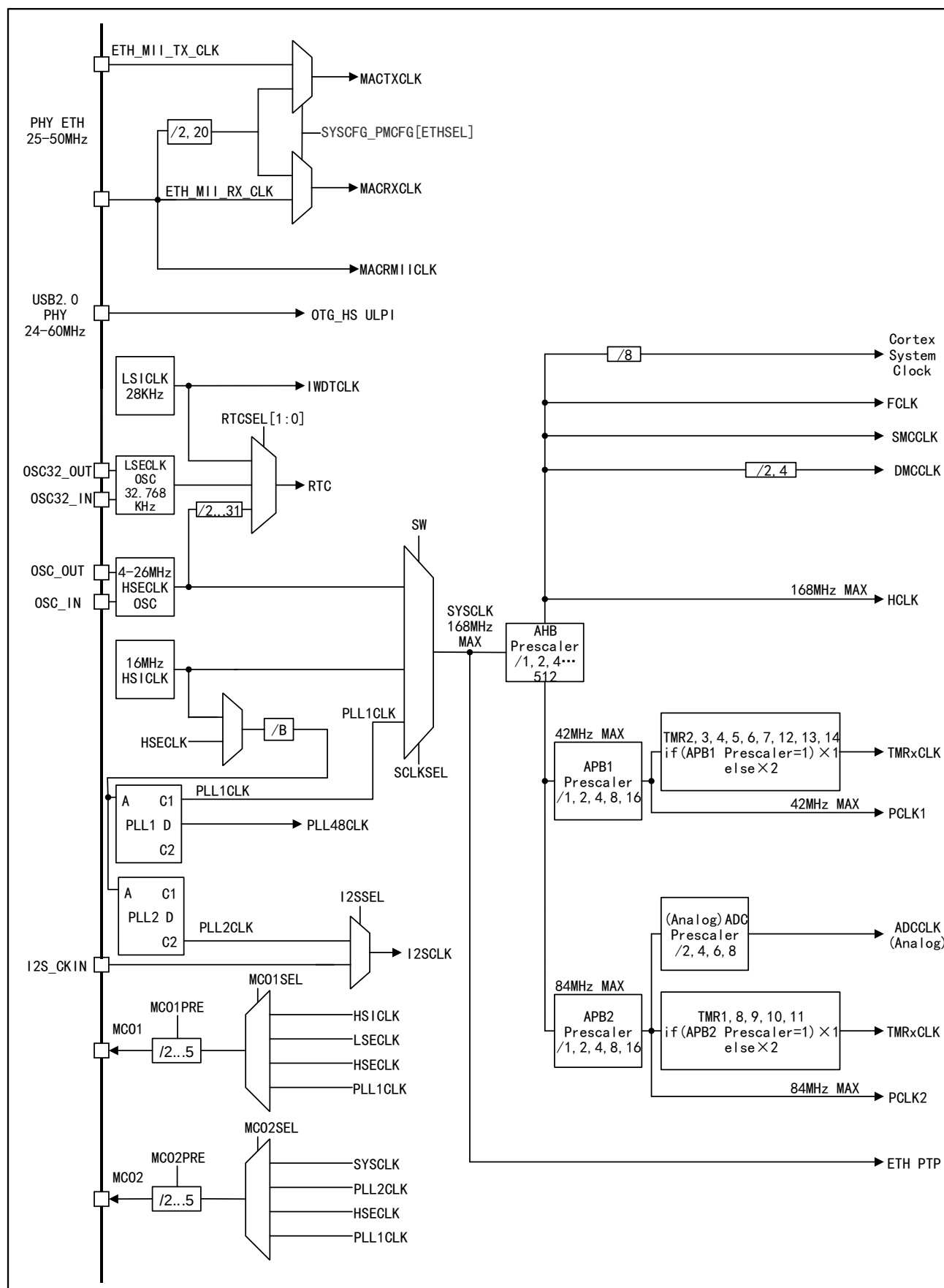
图 7 APM32F415xG 417xExG 时钟树
