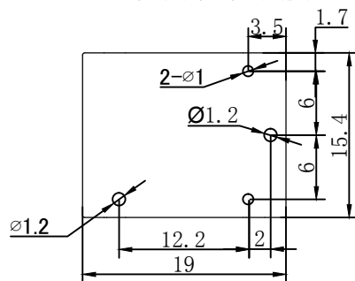
安装孔尺寸 (底视图)
