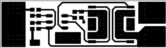
TOP SIDE
