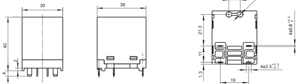
外形图
