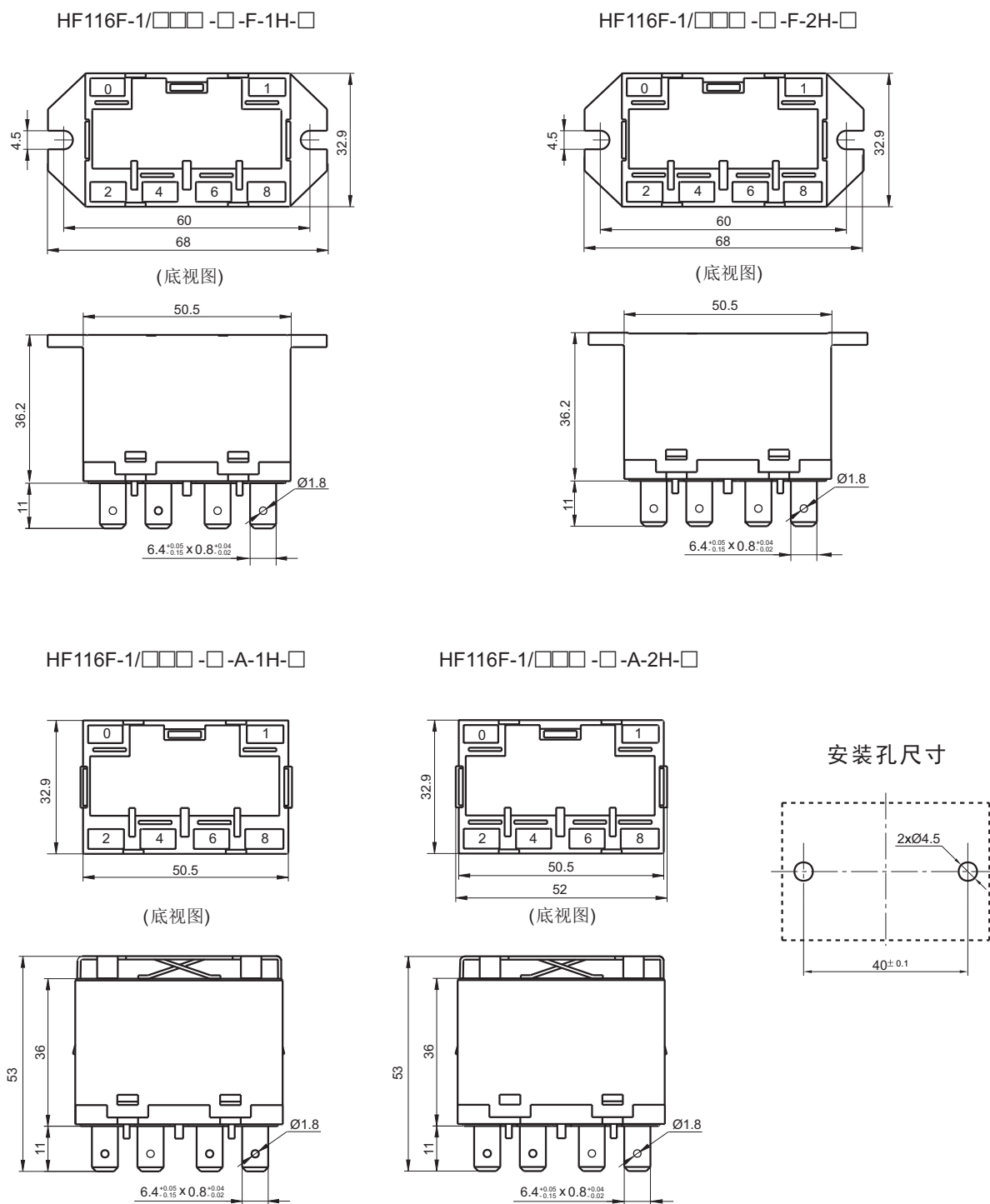
外形图
