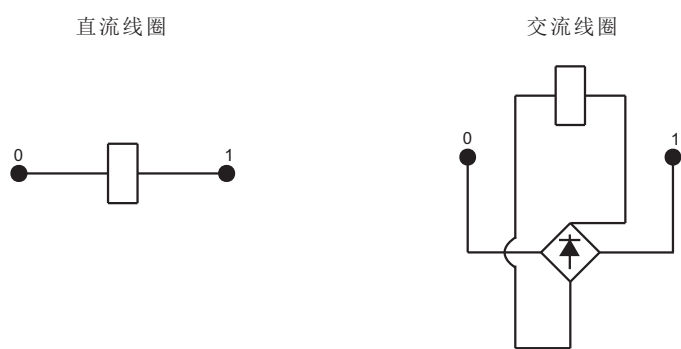
线圈接线图
