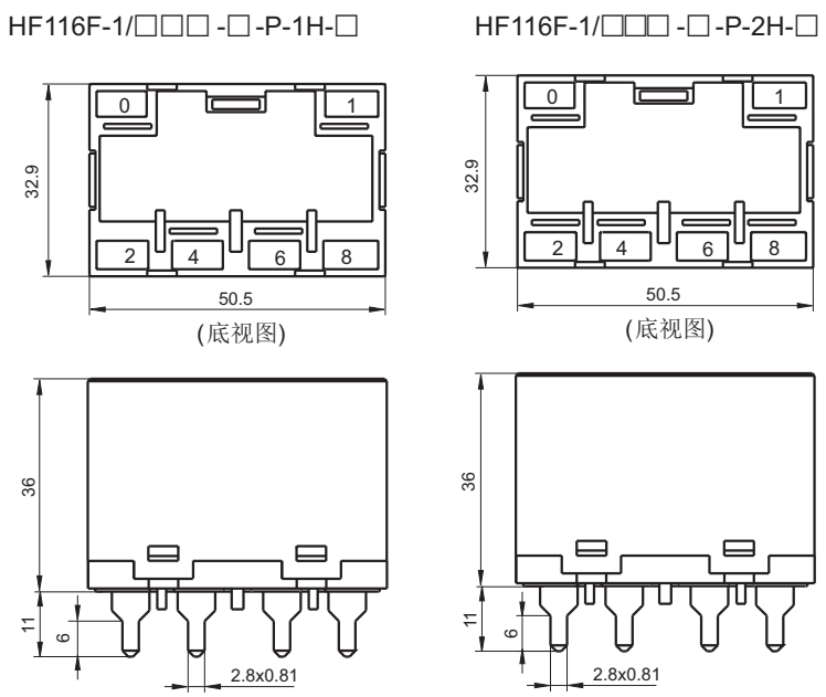
外形图
