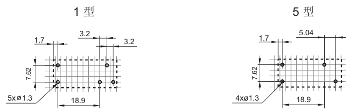
安装孔尺寸(底视图)
