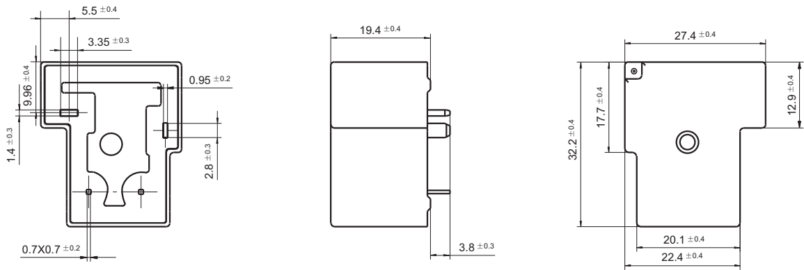
外形图
