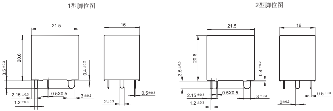
外形图
