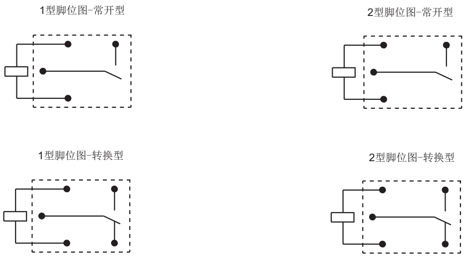
接线图(底视图)
