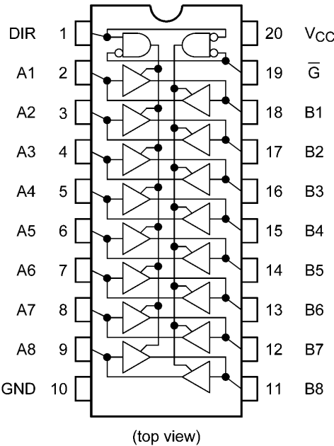
TC74AC245FT
