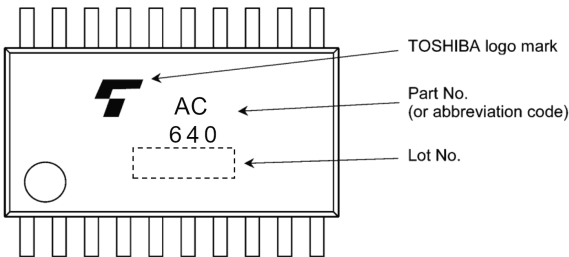
TC74AC640FT
