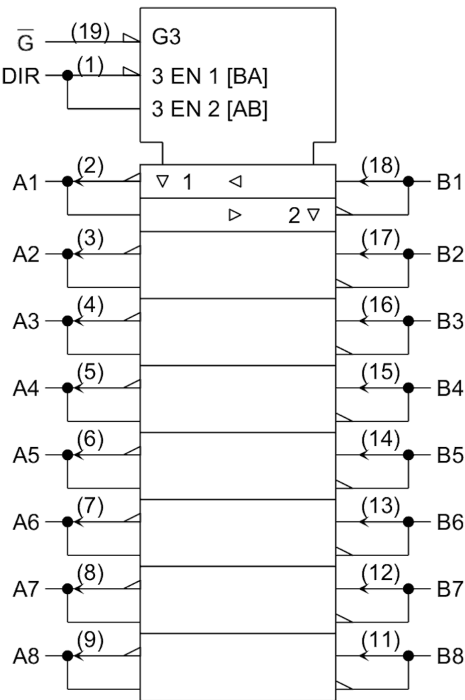
TC74AC640FT
