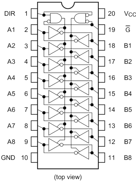
TC74AC640FT
