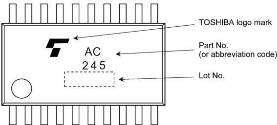
TC74AC245FT
