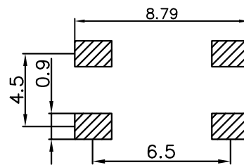
安装参考图
