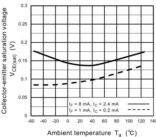
Fig. 11.10 V_{CE(sat)} - T_a
