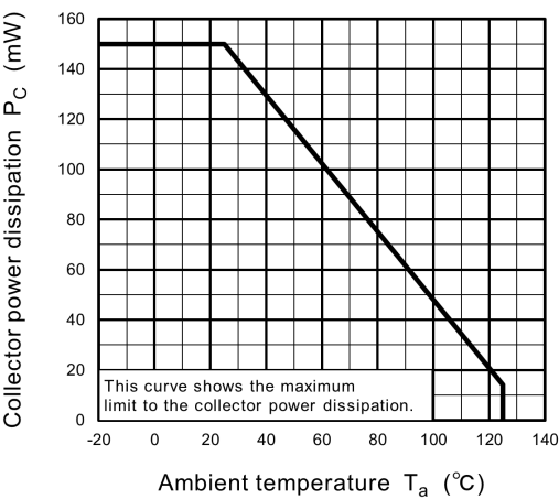
Fig. 11.2 P_C - T_a
