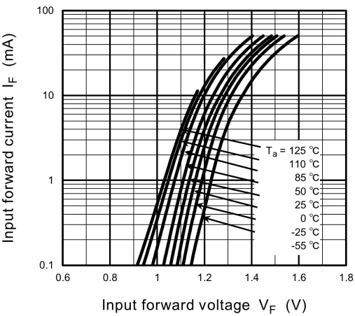
Fig. 11.4 I_F - V_F
