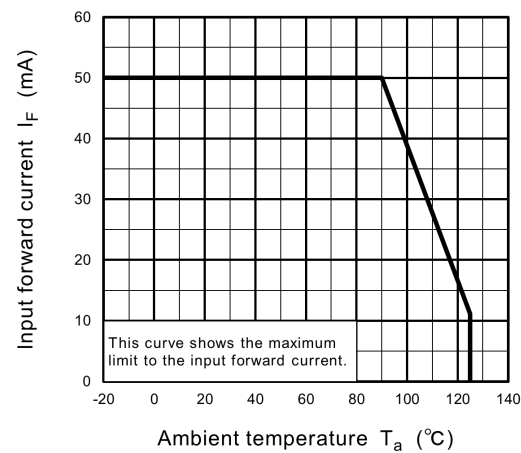
Fig. 11.1 I_F - T_a
