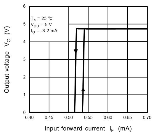
Fig. 13.2.10 V_O - I_F
