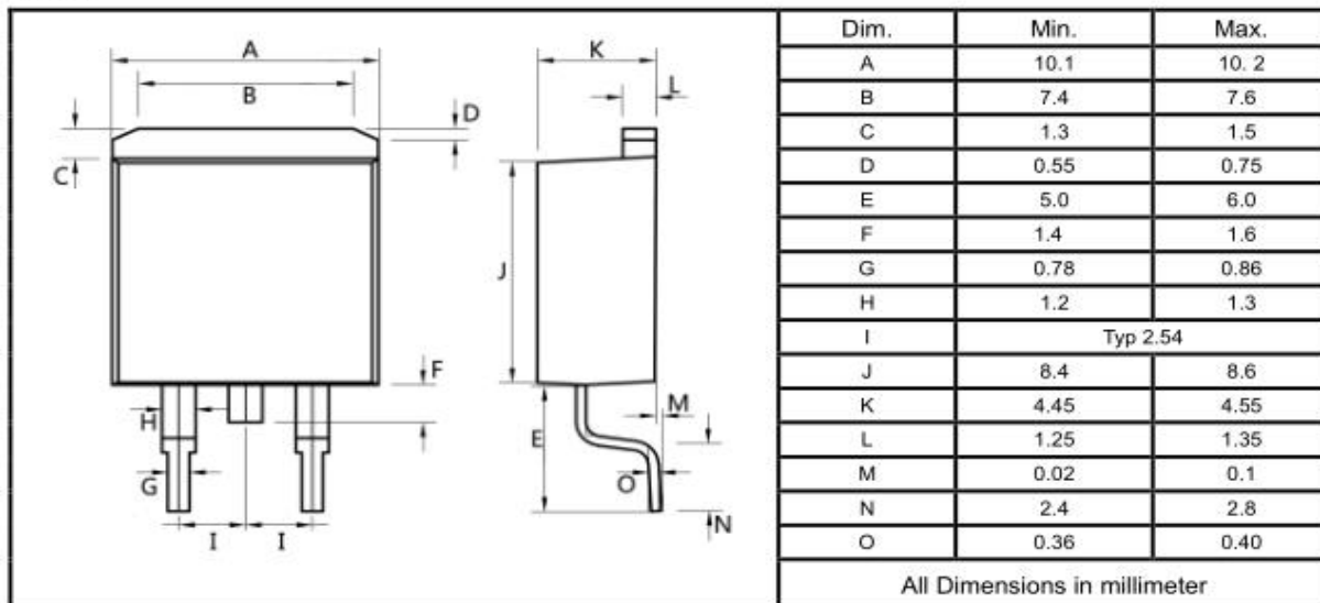
TO-263
