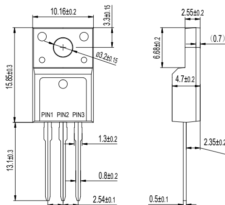
ITO-220AB
