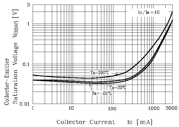
Fig. 4 V_{CE(sat)} - I_C
