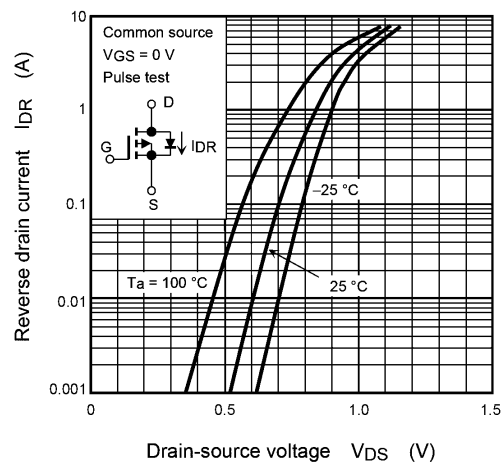
Fig. 8.8 I_{DR} - V_{DS}
