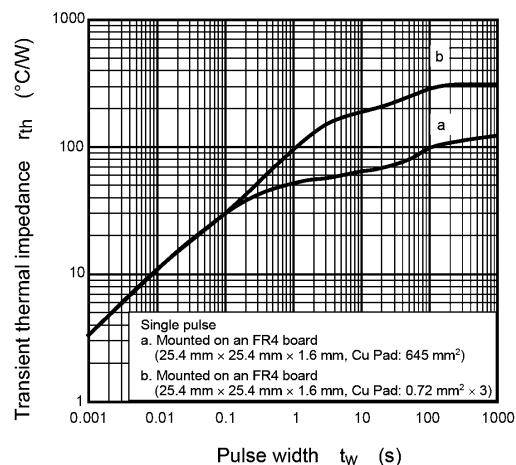
Fig. 8.12 r_{th} - t_w
