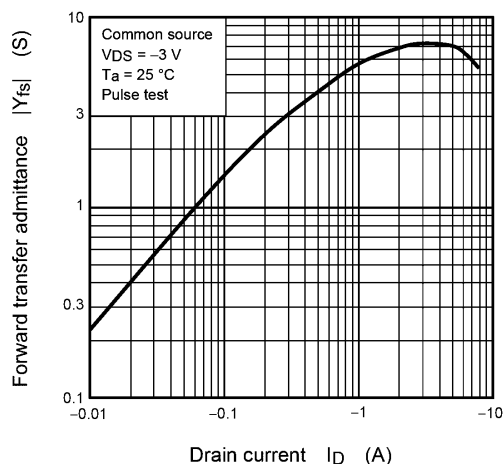
Fig. 8.7 |Y_{fs}| - I_D
