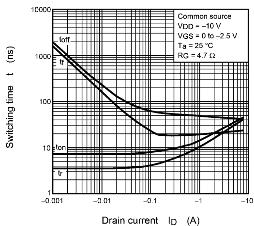
Fig. 8.10 t - I_D
