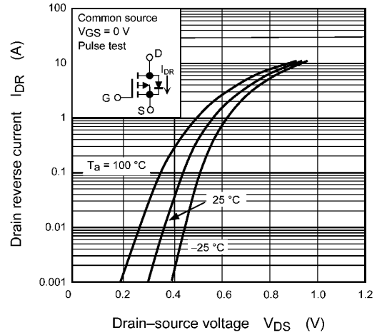
Fig. 7.8 I_{DR} - V_{DS}
