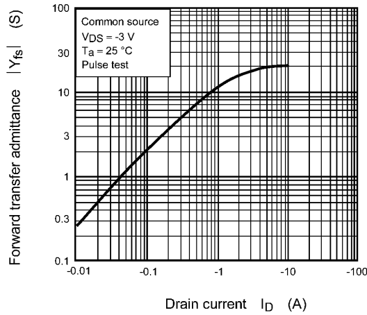
Fig. 7.7 |Y_{fs}| - I_D
