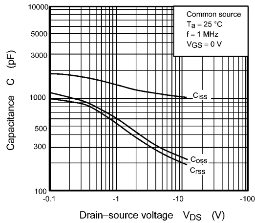
Fig. 7.9 C - V_{DS}
